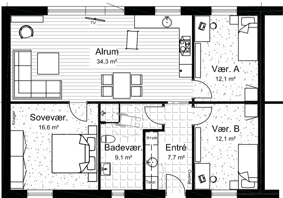
Princip for planindretning i bolig 1:100 Grundende er beliggende syd for Omme Landevej
